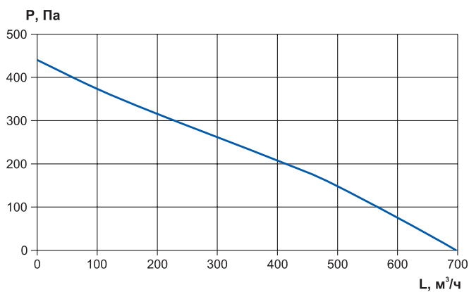
CV-SH-250-AC
