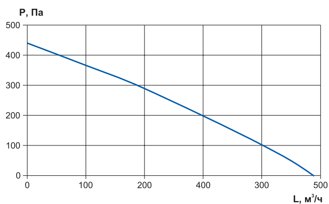
RWN-F-250-AC
