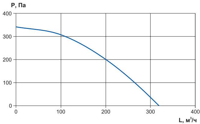
CV-SH-160-AC
