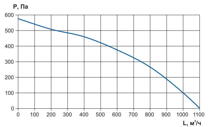
CV-SH-315-AC
