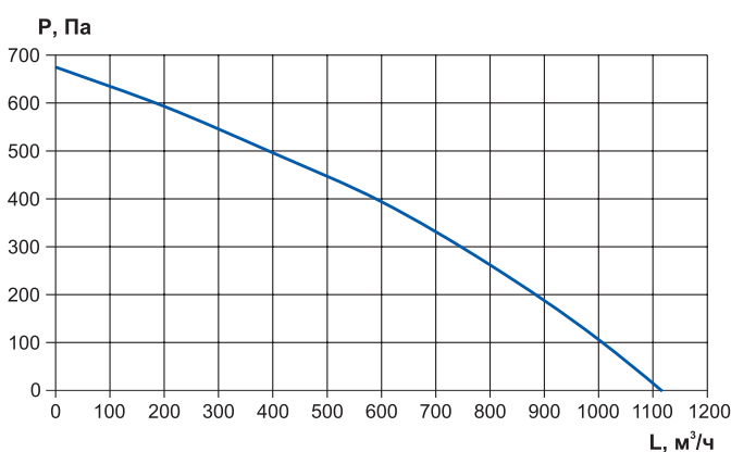
RWN-F-600-AC
