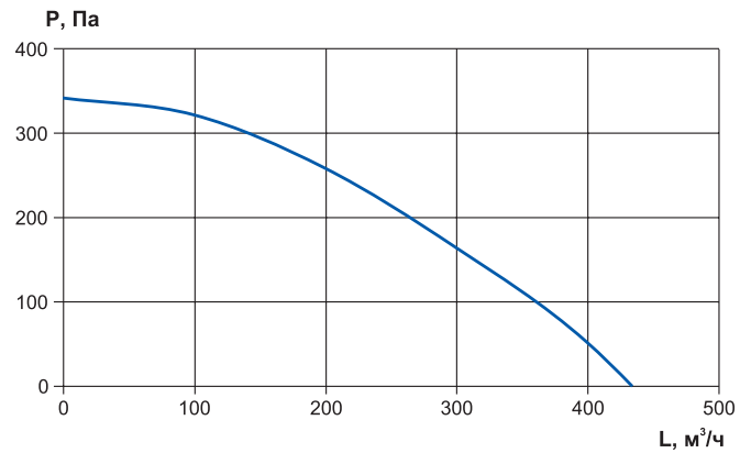
CV-SH-200-AC
