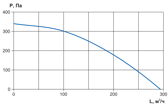
RWN-F-250-AC
