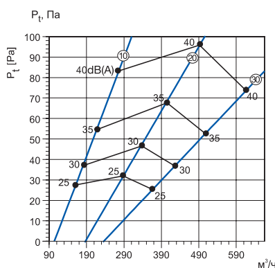
SRC 200-P
