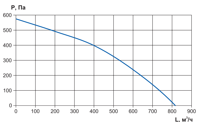
RWN-F-500-AC
