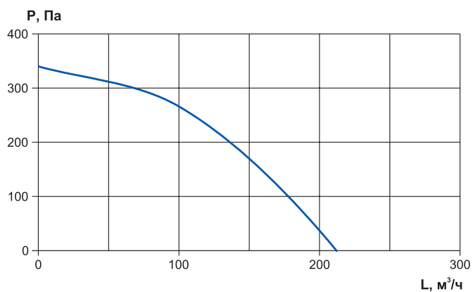
RWN-F-200-AC
