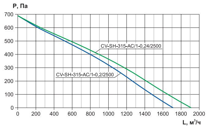
CV-SH-315-AC
