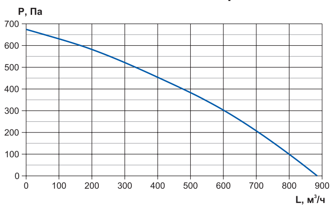
RWN-RP-800-AC-Compact
