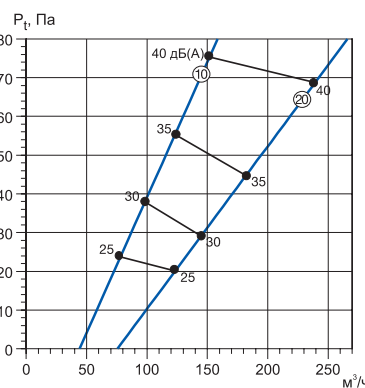
SRC 125-P
